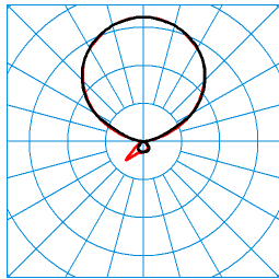
LuceoS S-T SMC PAW-IL 300-840 ETDI 05 (LEO2) TX369930 ■ C0 - C180 ■ C90 - C270 DIN 5040: E03 UTE: 0,08 D + 0,91 T CEN Flux Code: 53 86 96 8 100 49 82 98 92
