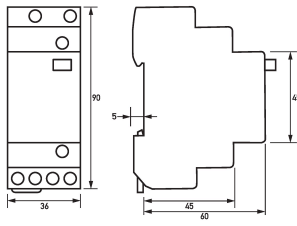
Maßzeichnung Gruppenansicht
