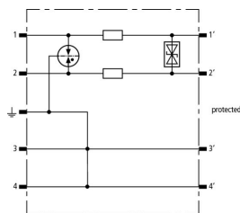
Prinzipialschaltbild BSP M2 BD HF 24
