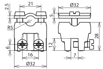
Maßbild FK ZS 7.10 KBF0.7 6 ZG
