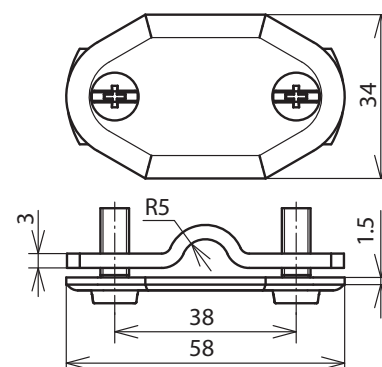
Maßbild NS 7.10 FL30 OZ AL
