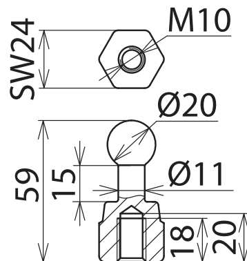
Maßbild KFP 20 M10
