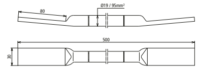
Maßbild
