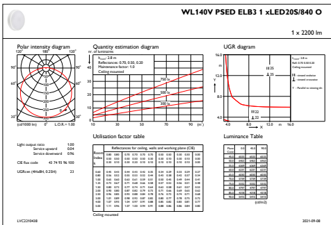
IFGU1_WL140VPSEDELB31xLED20S840O
