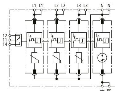
Prinzipschaltbild DG MP TT 275 FM
