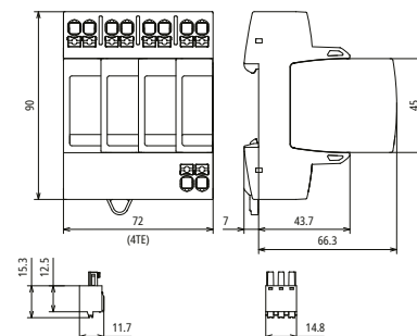
Maßbild DG MP TT 275 FM
