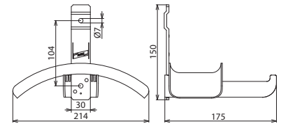
Maßbild HV EKV ES30 1500
