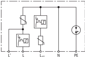
Prinzipschaltbild DEHNcord
