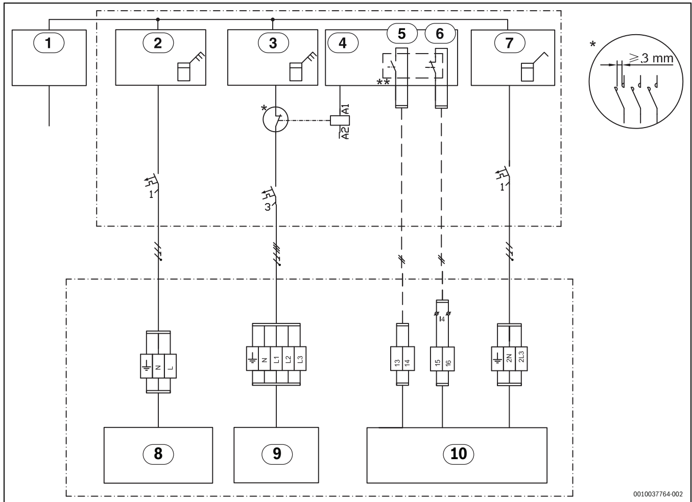
Bild 53 EVU Typ 3
