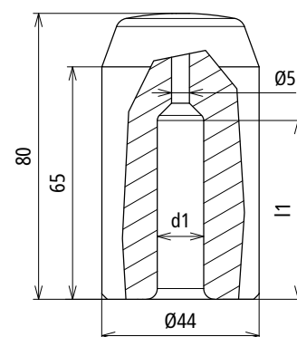
Maßbild SKO TE 20 STBLANK
