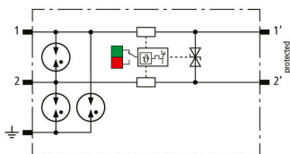
Prinzipialschaltbild BCO CL2 BD EX 24
