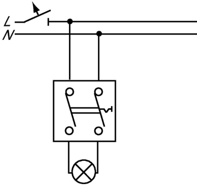
Anschlussbild
