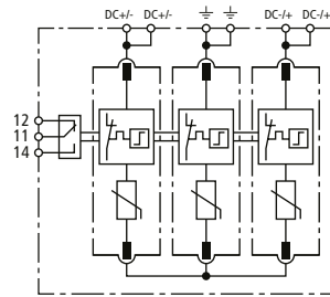
Prinzip Schaltbild
