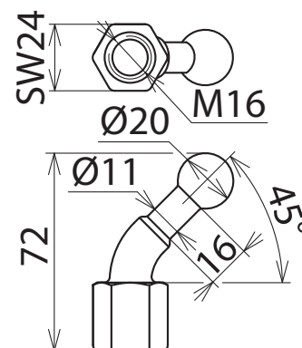
Maßbild KFP 20 W45 M16
