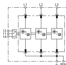
Prinzipialschaltbild DV M2 TNC 255 FM
