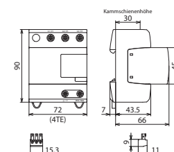
Maßbild DV M2 TNC 255 FM
