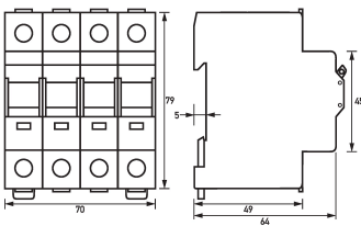
Maßzeichnung Gruppenansicht
