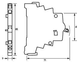
Maßzeichnung Gruppenansicht
