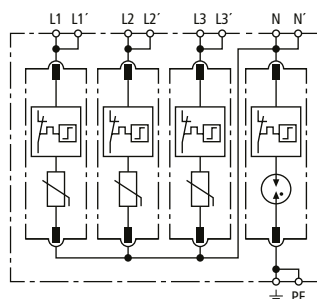
Prinzipschaltbild DG MP TT 275
