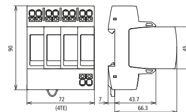
Maßbild DG MP TT 275
