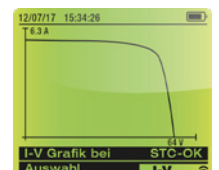
Ergebnisse können grafisch als I-U Kennlinie dargestellt werden, inkl. auto. Auswertung OK / Nicht OK
