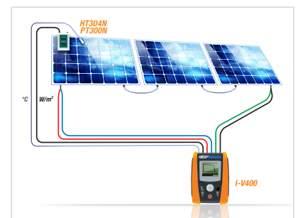
Anschluss I-V400w direkt an HT304
