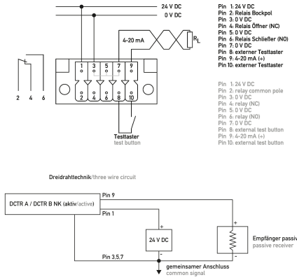
Anschlussschema Pinbelegung zehnpolige Steckbuchse (spannungslos)
