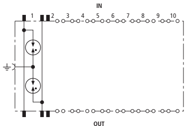
Prinzipschaltbild DPL 10 G3 110 FSD
