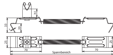
Maßbild DLH SG 8 H20 FG180.280 V2A
