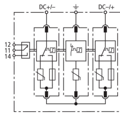
Prinzipschaltbild DG M YPV SCI 150 FM
