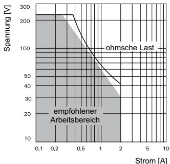
Lastkurve der Signalrelais (AC/DC)
