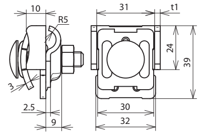
Maßbild FK KB 6.10 KBF0.7 8 AL
