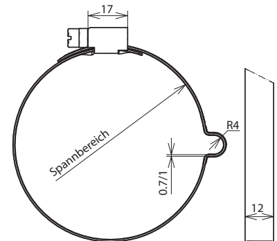
Maßbild LH 8 SB100.120 SCG V2A
