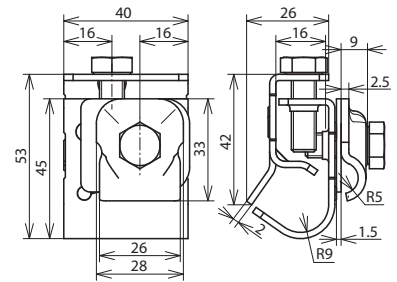
Maßbild ZMDRK KB 6.10 W16.22 CU STTZN
