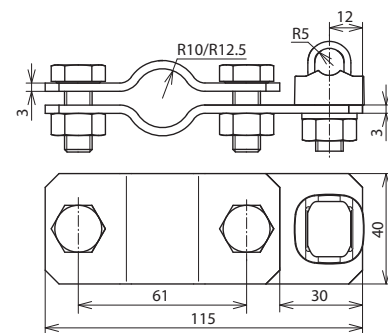
Maßbild AS TE 20 KSV 7.10 STTZN
