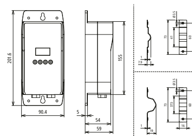
Maßbild DLSC 100
