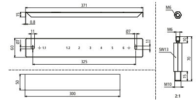
Maßbild
