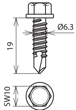
Maßbild BSC 6.3X19 SW10 V2A
