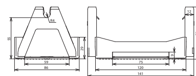
Maßbild DLH KF2 8 LO 141X86X70
