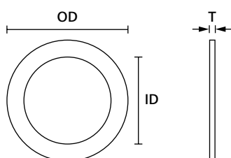
HelaGuard Dichtungsscheibe
