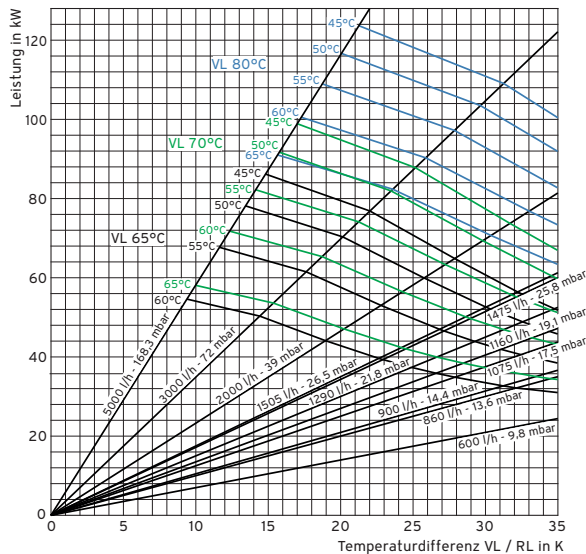
Leistungdiagramm VIH SW 500
