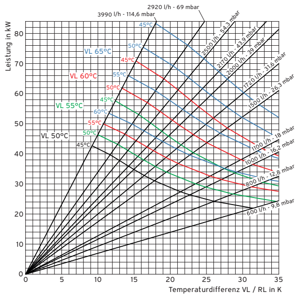
Leistungdiagramm VIH SW 500
