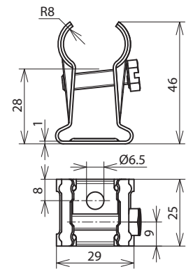
Maßbild SH KR 13.16 H28 B6.5 V2A
