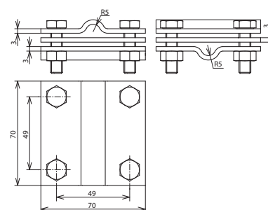
Maßbild KS 7.10 7.10 FL40 ZP V4A
