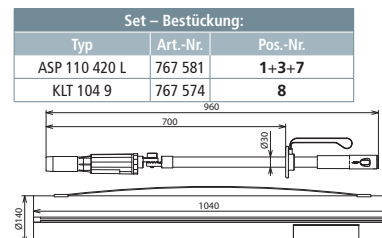
Maßbild ASPS 110 420 L
