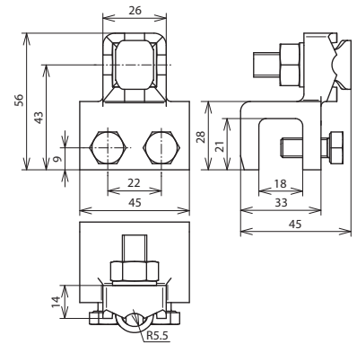
Maßbild AK 7.10 KSV KBF8 18 TGTZN
