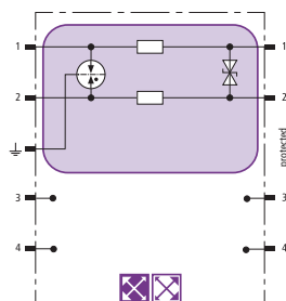
Prinzipschaltbild BXT ML2 BD 180
