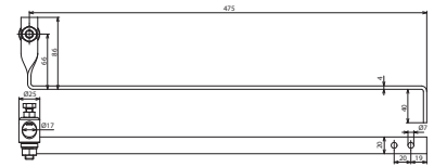
Maßbild SH BB16 L475 WS V2A STTZN
