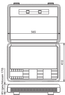
Maßbild KK 56 41 17 EK VI TI
