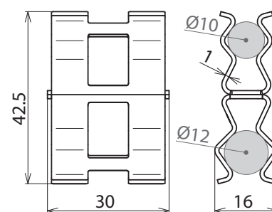
Maßbild DC BK 12 RD10 STBLANK
