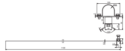
Maßbild BS D50 DS30 SB50.300 V2A
