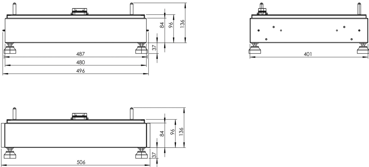
Abbildung 9. Abmessungen — Sockel
