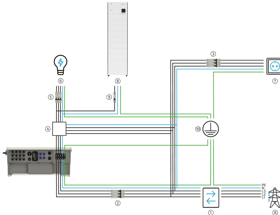
Abbildung 22. AC-Anschluss allgemein
