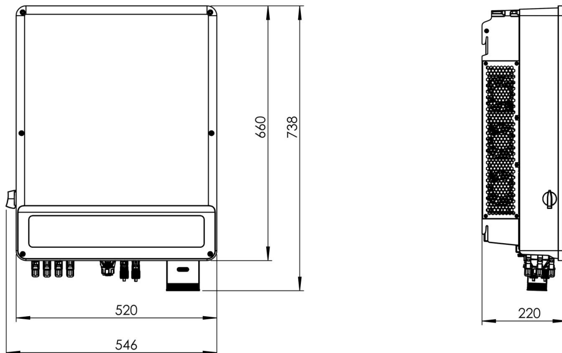
Abbildung 1. Wechselrichter — Abmessungen
