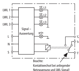
Prinzipialschaltbild DSI E 3
