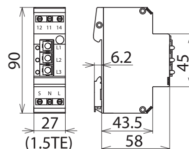
Maßbild DSI E 3
