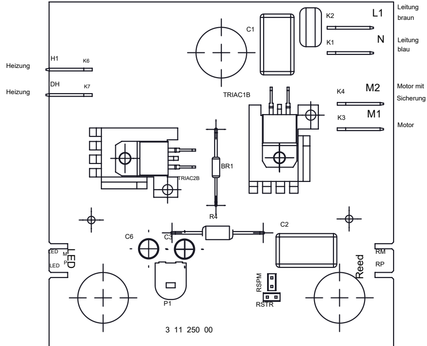
Schaltplan Elektronik AirStar TB-C1
