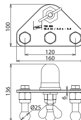
Maßbild EAPA 3 KFP 25 KKH
